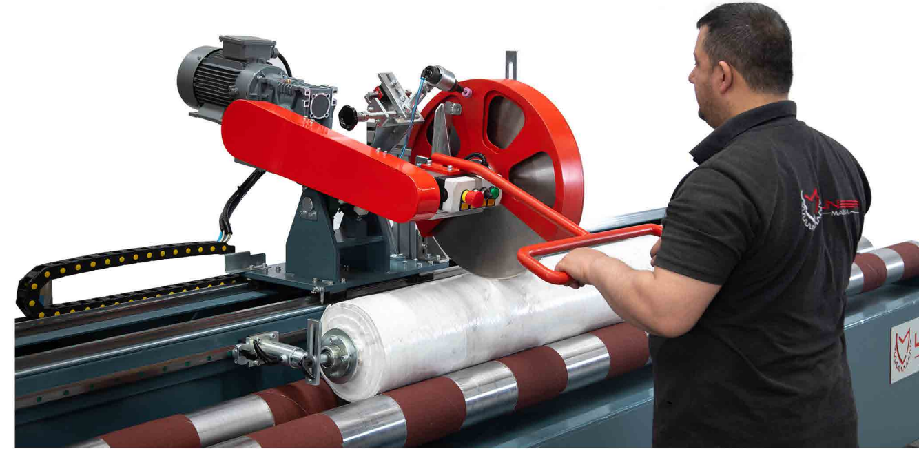
Rulo Tutucu Apara
